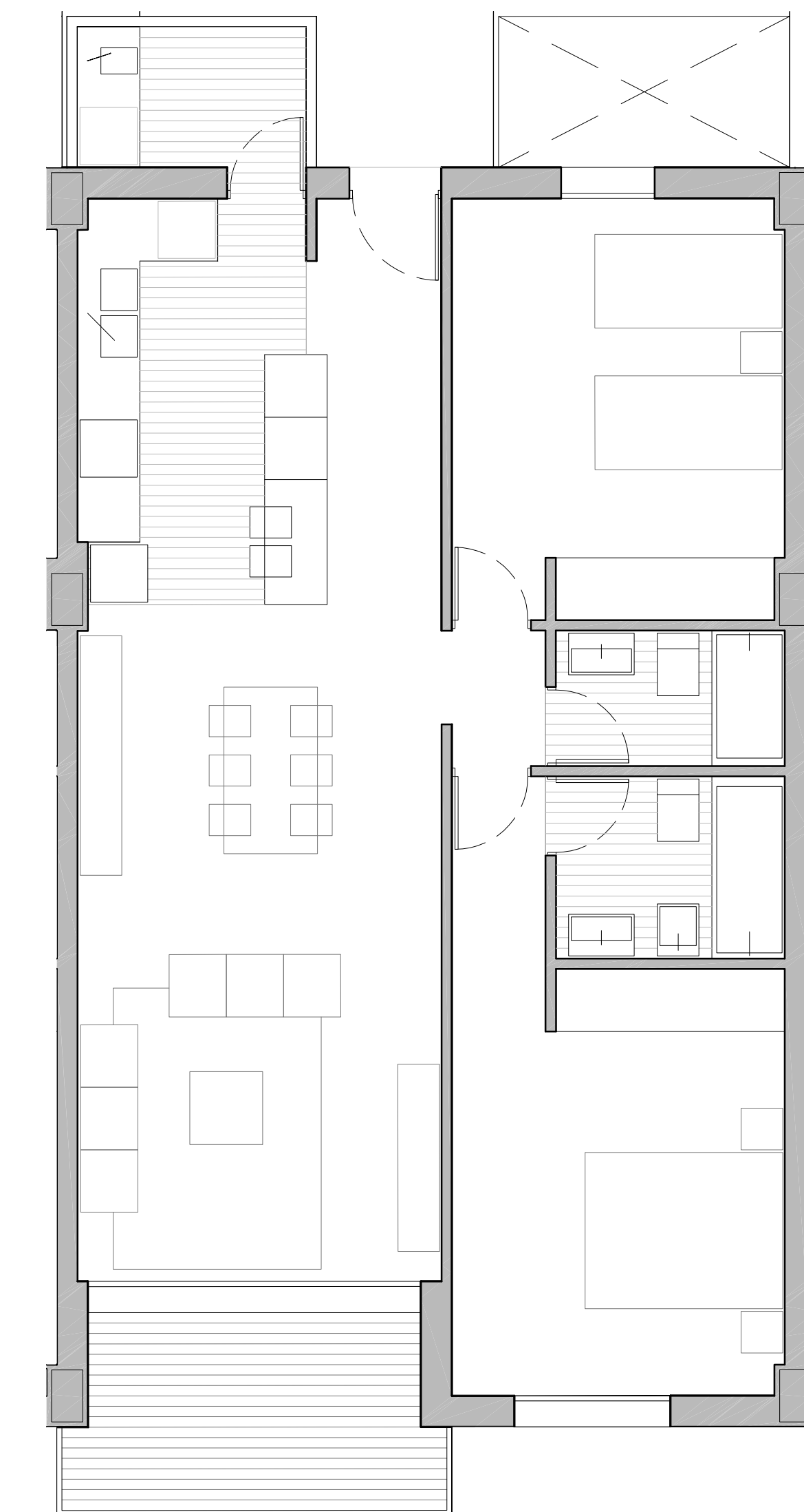
PLANTA PRIMERA
