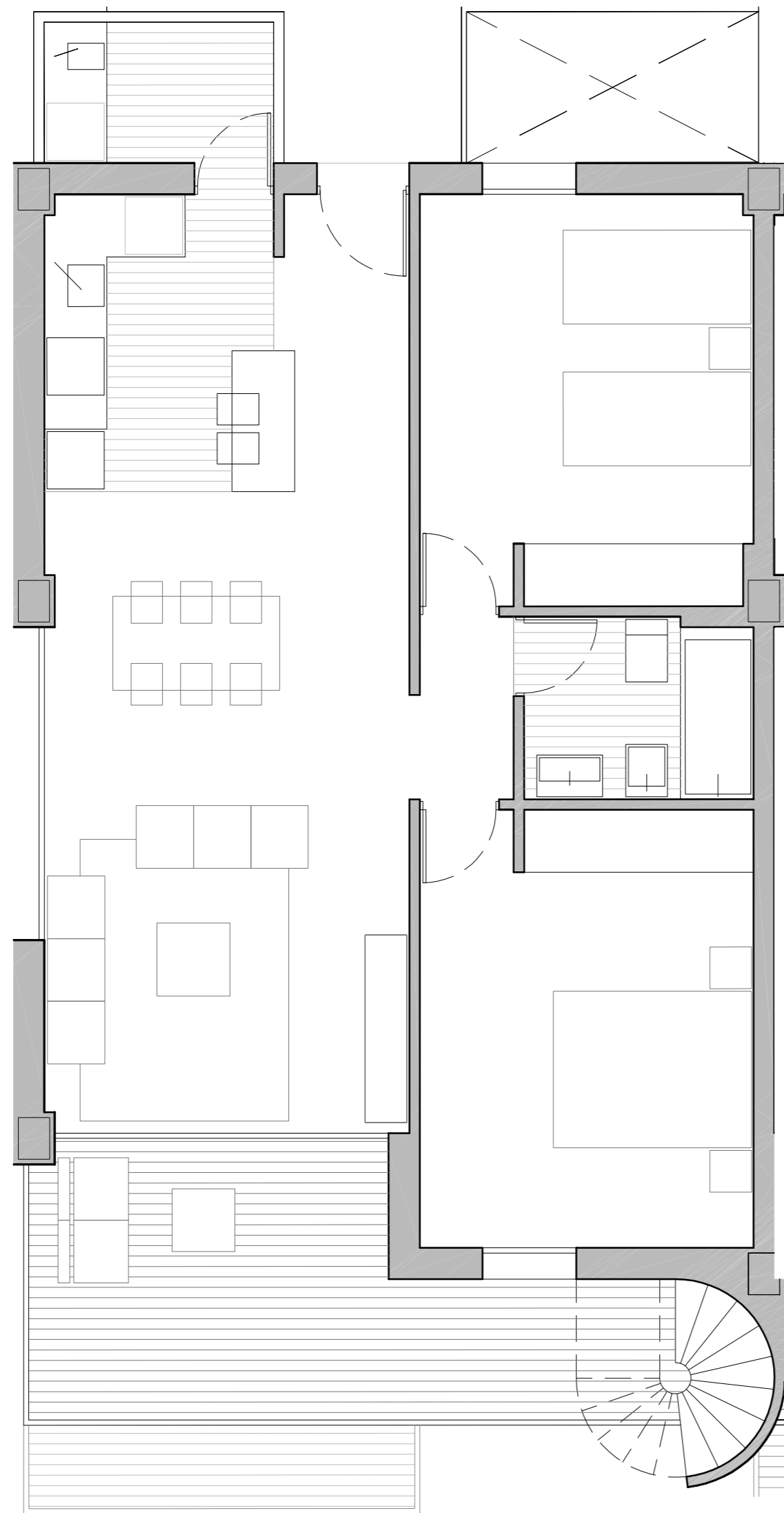
PLANTA SEGUNDA
