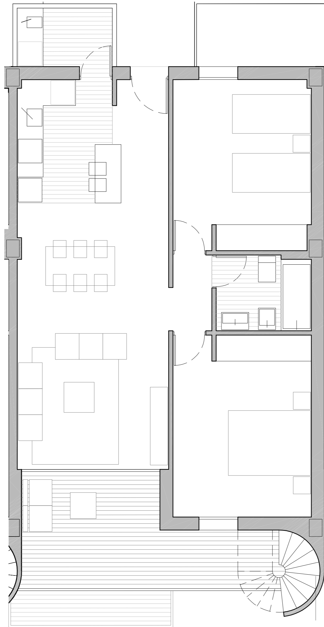
PLANTA SEGUNDA
